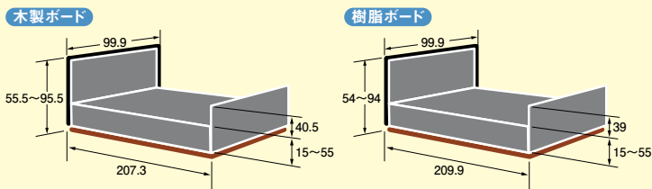
寸法表
