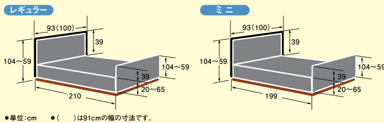
寸法表
